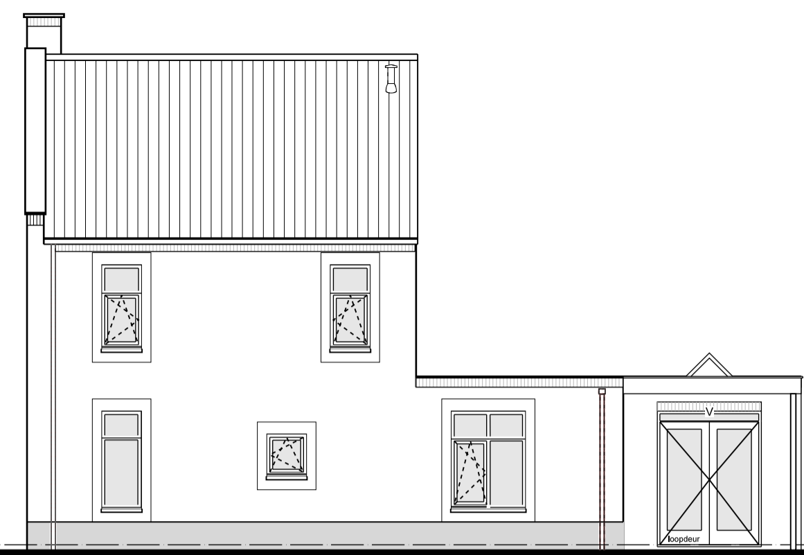
RECHTER ZIJGEVEL OPTIE: TERRAS OVERKAPPING ACHTERGEVEL
