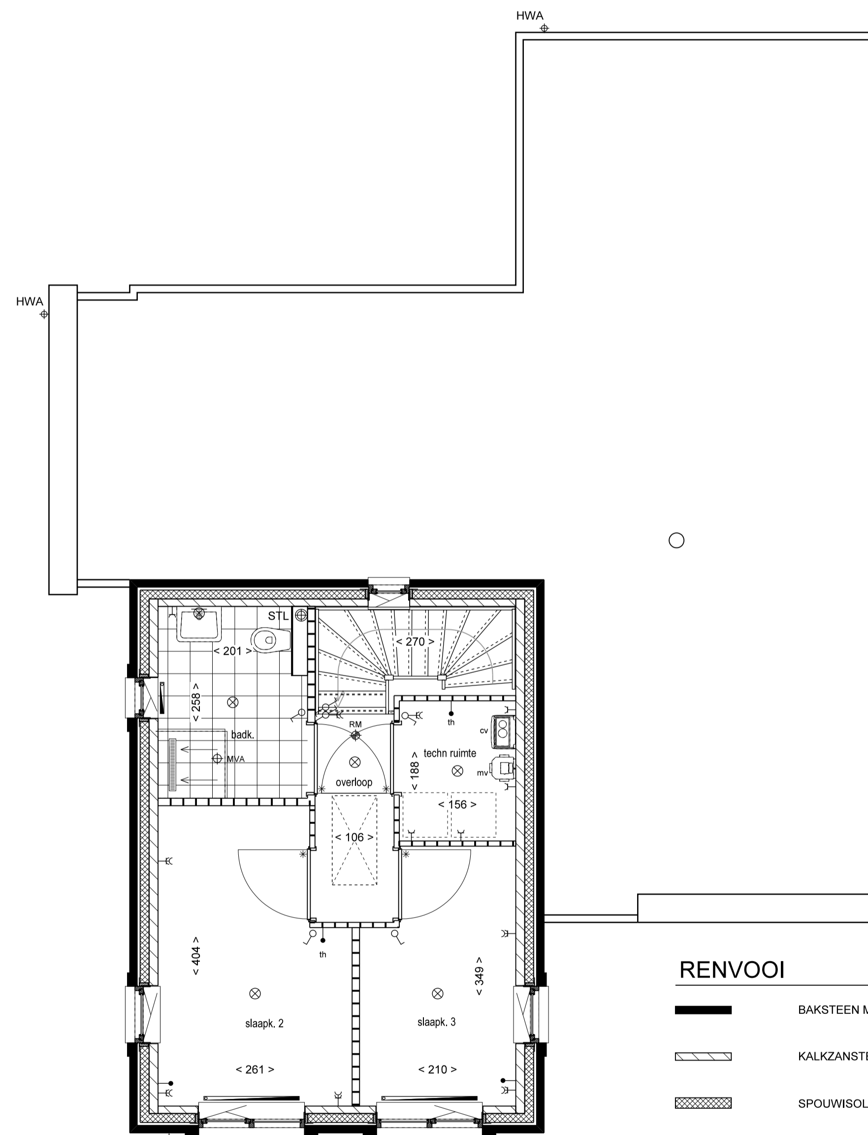
1e VERDIEPING TYPE L2
