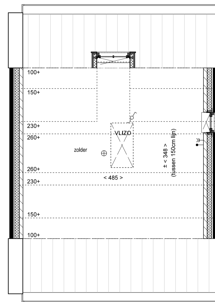
2e VERDIEPING TYPE L2
